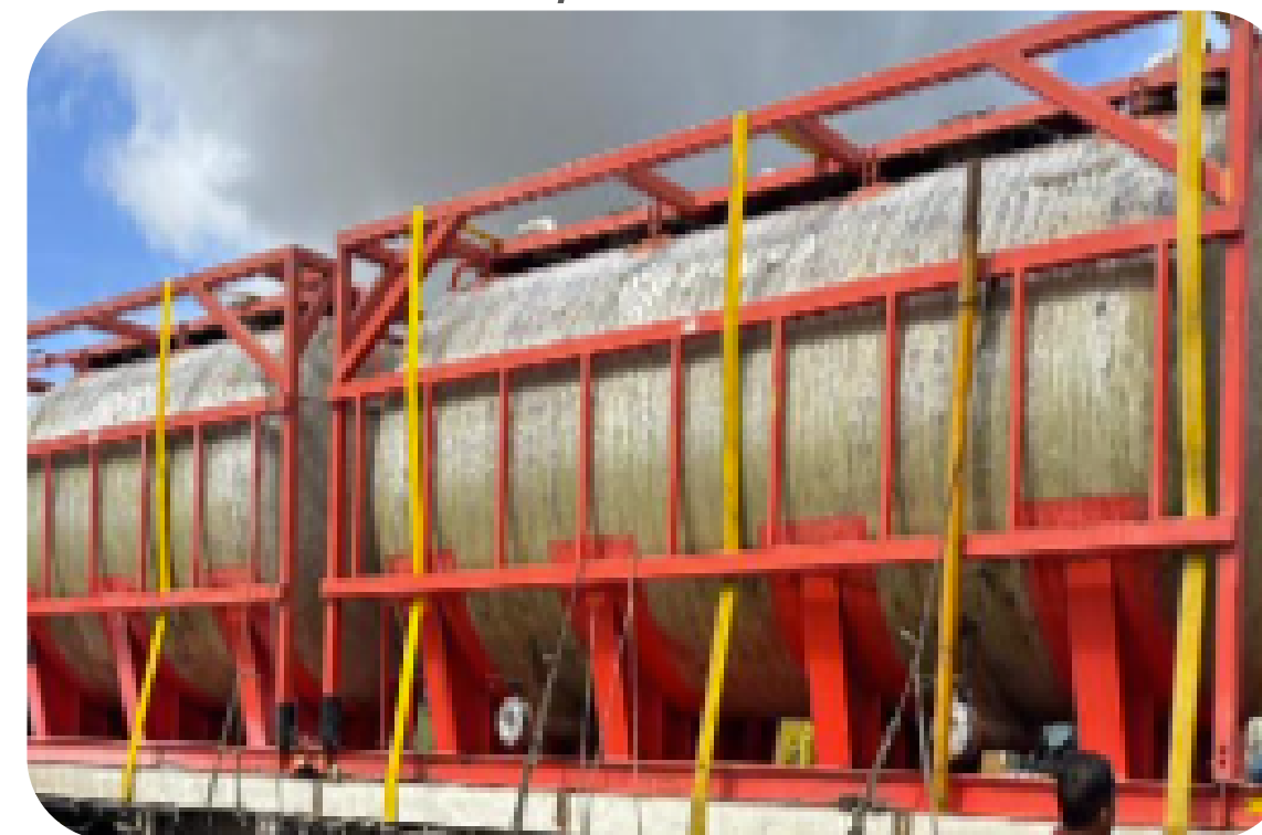
TANQUE DE DESPLAZAMIENTO PDV-TC-TD-15-1 / PDV-TC-TD-15-2
